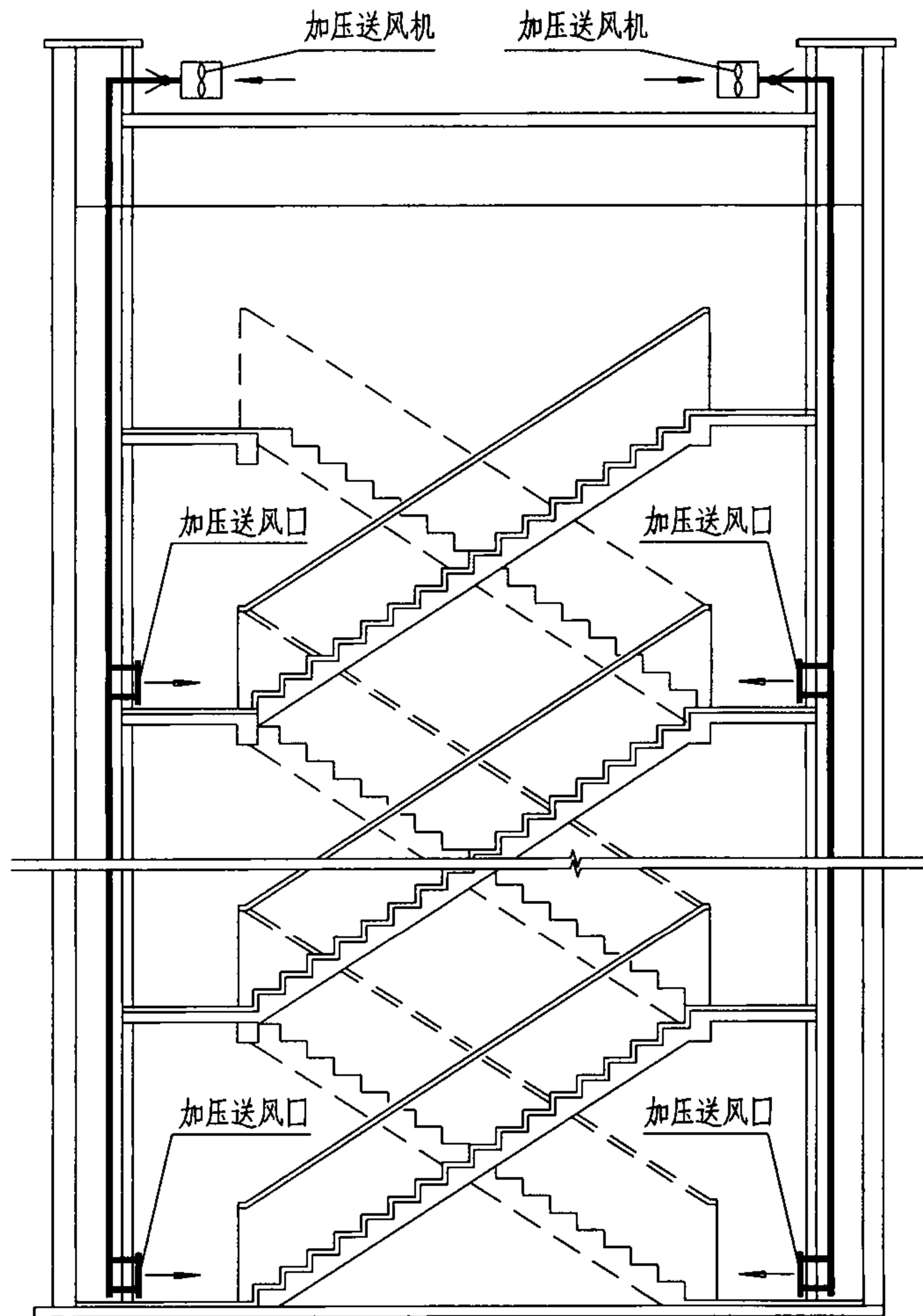
A-A剖面图
